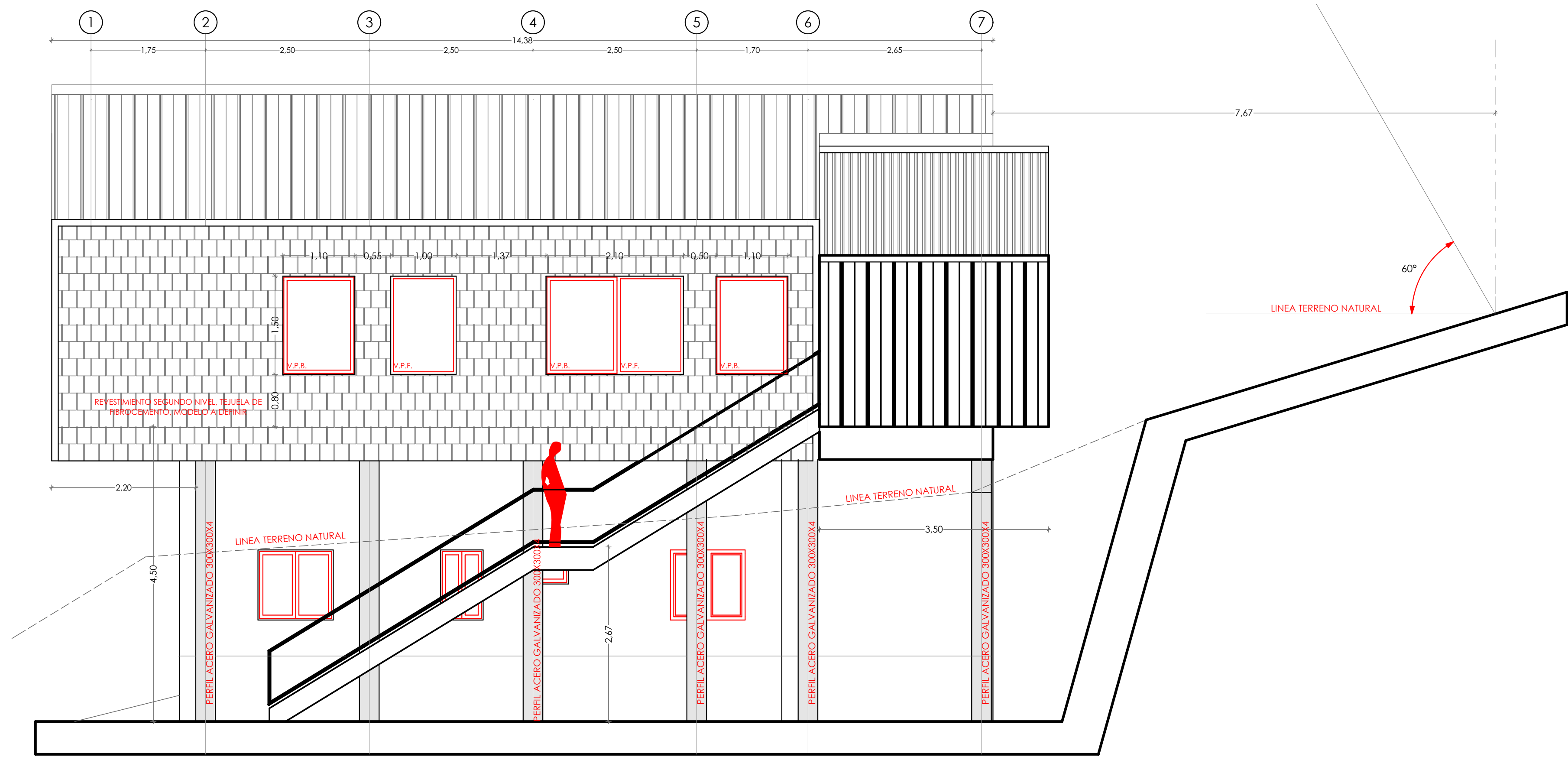
ELEVACIÓN LATERAL DERECHA esc 1:50
