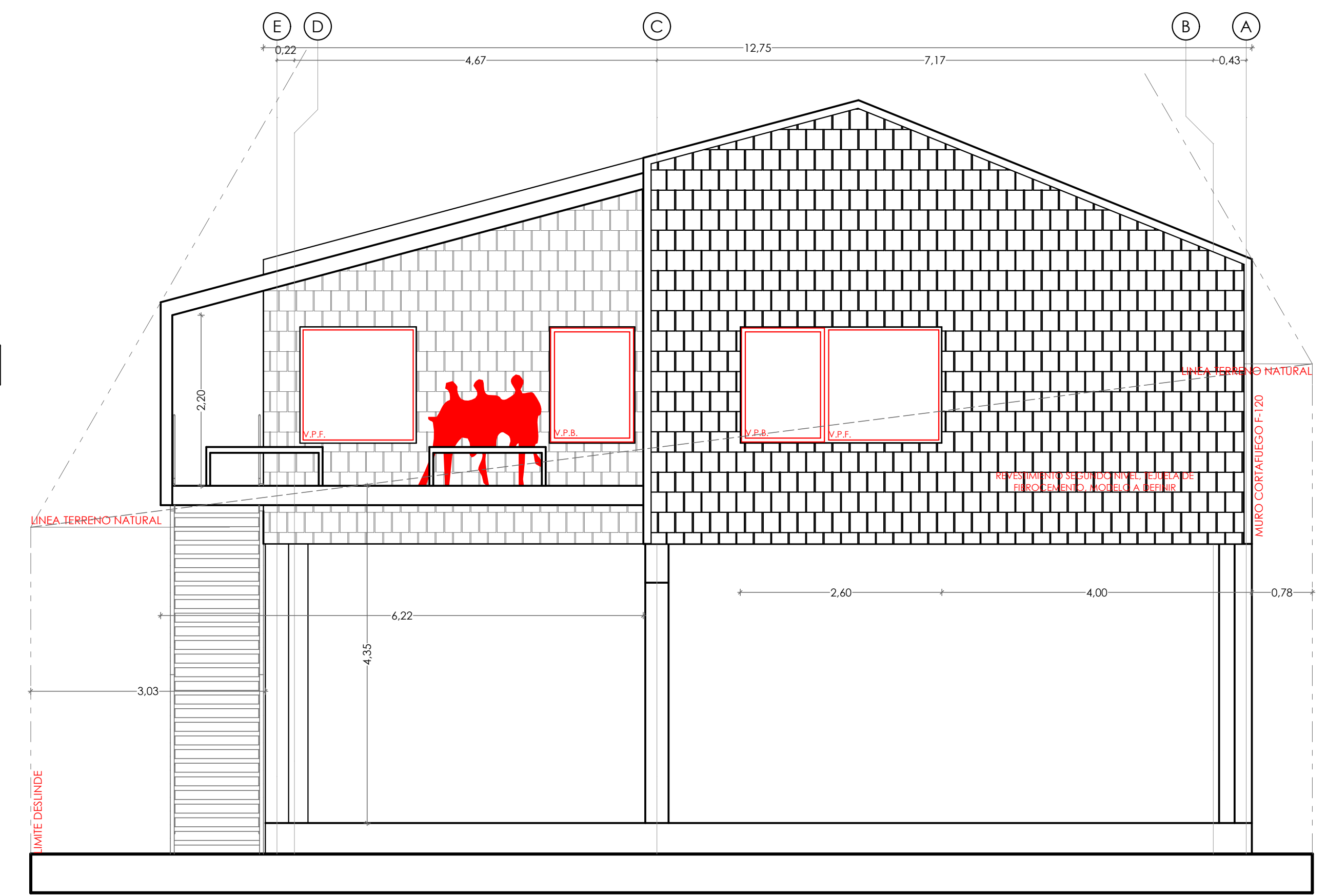
ELEVACIÓN POSTERIOR esc 1:50
